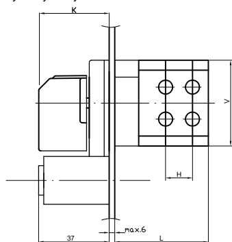
S 63, 80, 100, 125, 160 JT
