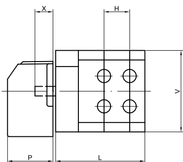
S 63, 80, 100, 125, 160 J
