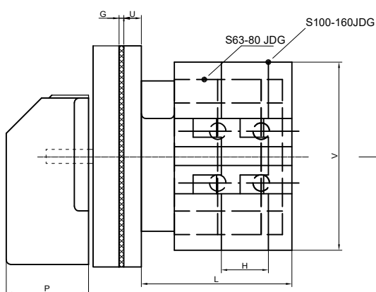
S 63,80, 100, 125, 160 JDG
