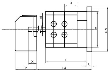
S 63, 80, 100, 125, 160 JO
