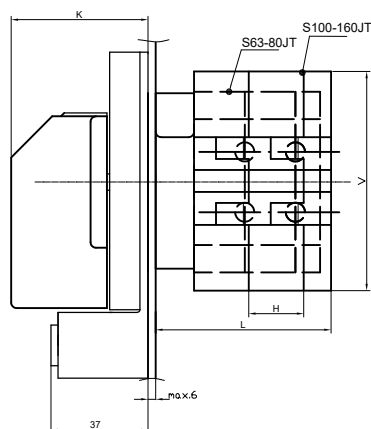
S 63, 80, 100, 125, 160 JT
