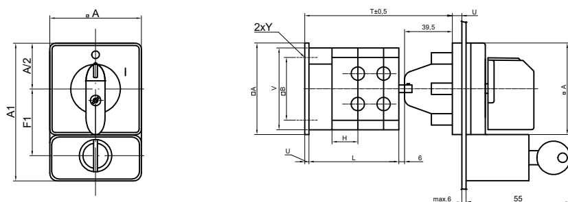
S 63, 80, 100, 125, 160 JBZ
