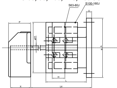
S 63, 80, 100, 125, 160 JO
