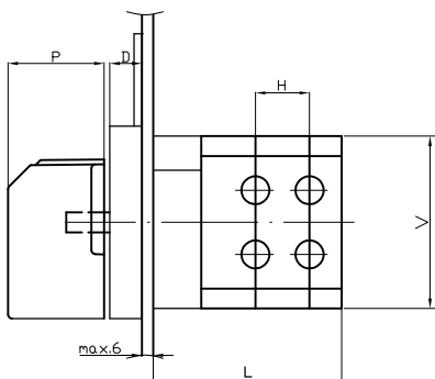
S 63, 80, 100, 125, 160 JD
