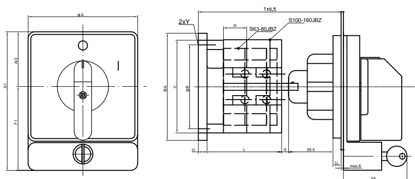
S 63, 80, 100, 125, 160 JBZ
