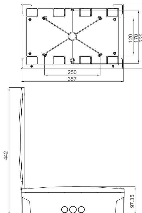
Распределительный щит P-Box над штукатуркой, 16 модулей
