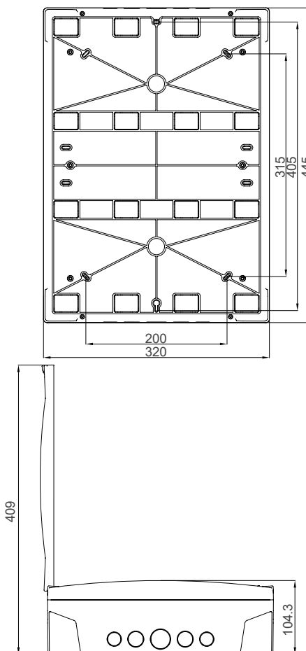
Распределительный щит P-Vox над штукатуркой, 36 модулей, тройной ряд
