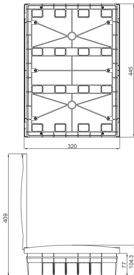
Распределительный щит P-Vox под штукатурку, 36 модулей, тройной ряд
