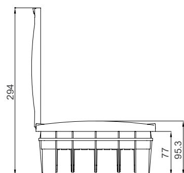
Распределительный щит P-Box под штукатурку, 12 модулей
