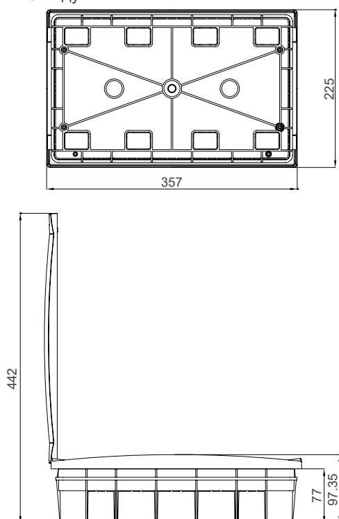
Распределительный щит P-Box под штукатурку, 16 модулей
