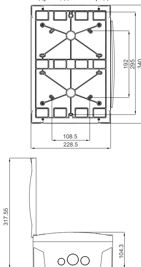
Распределительный щит P-Box над штукатуркой, 16 модулей, двойной ряд
