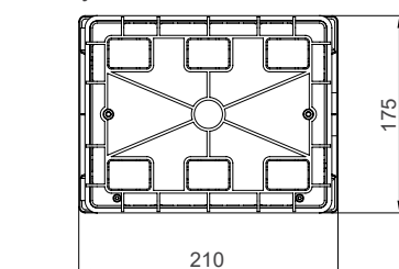
Распределительный щит P-Box под штукатурку, 8 модулей
