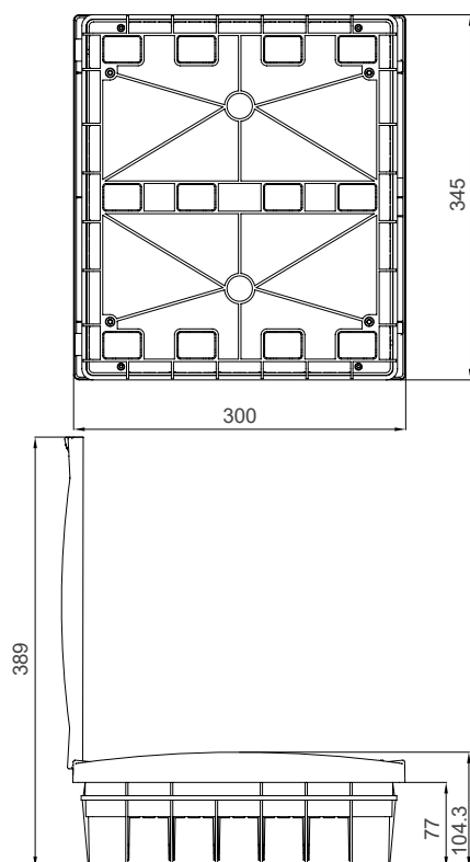
Распределительный щит P-Vox под штукатурку, 24 модулей, двойной ряд
