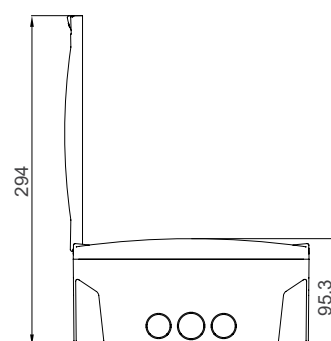
Распределительный щит P-Box над штукатуркой, 12 модулей
