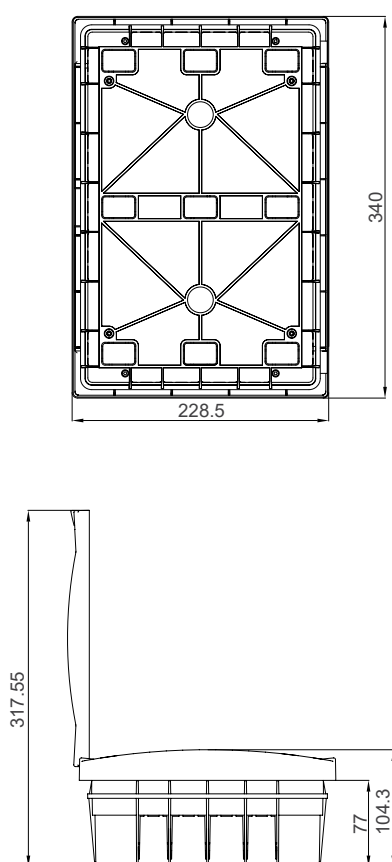
Распределительный щит P-Box под штукатурку, 16 модулей, двойной ряд
