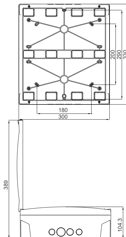
Распределительный щит P-Vox над штукатуркой, 24 модулей, двойной ряд
