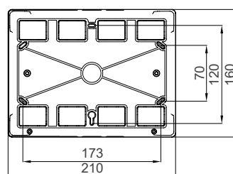
Распределительный щит P-Box над штукатуркой, 8 модулей
