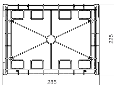
Распределительный щит P-Box под штукатурку, 12 модулей
