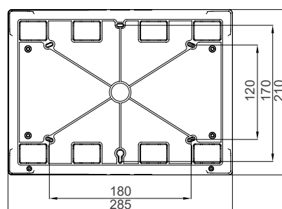
Распределительный щит P-Box над штукатуркой, 12 модулей
