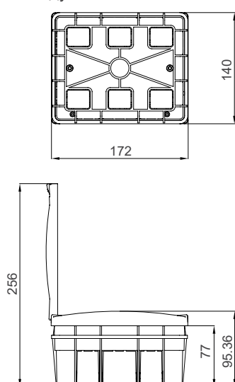
Распределительный щит P-Vox под штукатурку, 6 модулей
