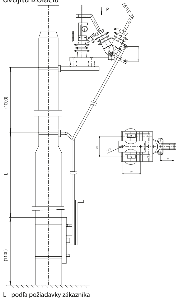
OMDI, OZTI s ručným pohonom dvojité izolácia
