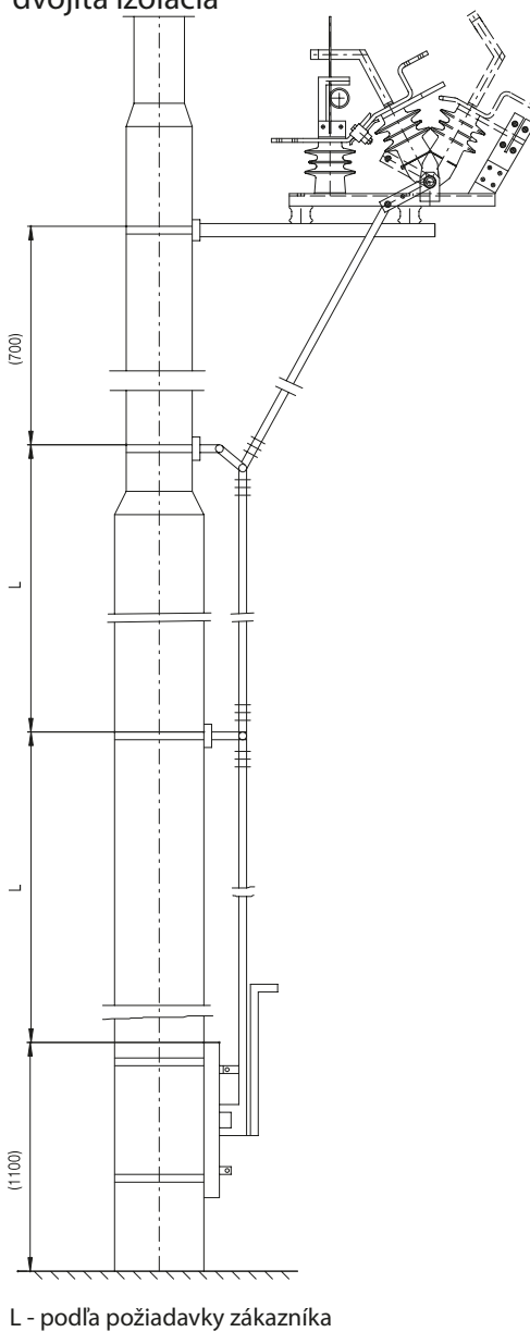
OMDZ, OZTZ s ručným pohonom dvojité izolácia
