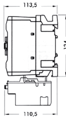
Rozmerový náčrt
