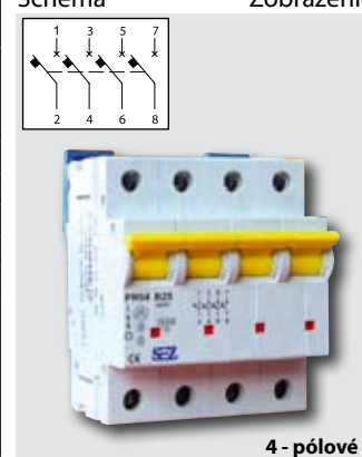
Schéma
